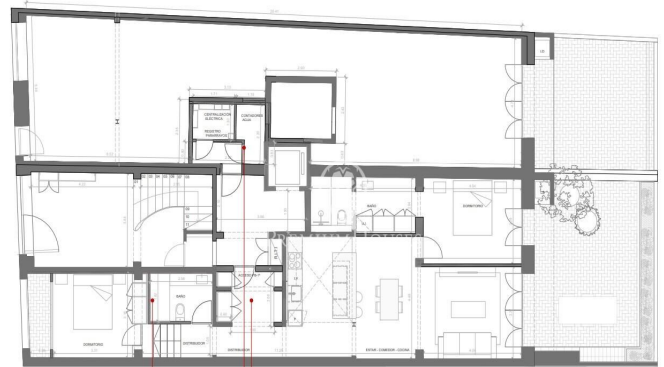
PLANTA SALA
