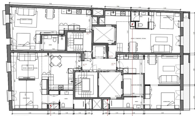
PLANTA TERCERA
