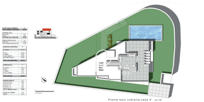
Planta bajo cubierta, casa K
