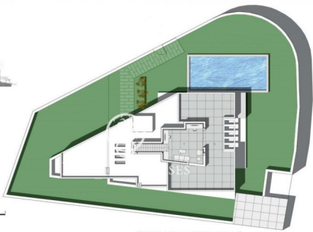
Planta bajo cubierta, casa K hdl. 1/100
