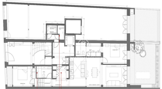
PLANTA SALA
