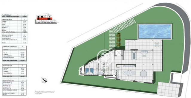
Planta baja, casa K m2: 1100
