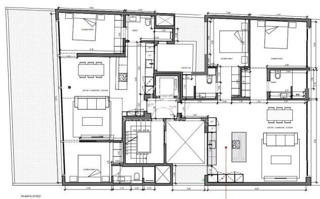
PLANTA CUARTA
