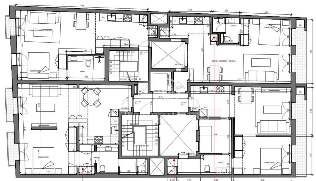
PLANTA SEGUNDA
