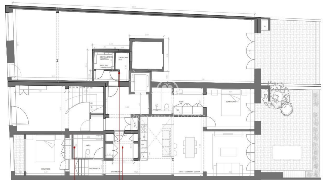
PLANTA SALA
