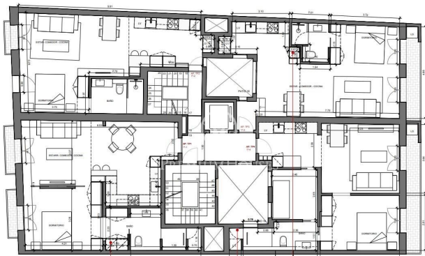
PLANTA PRIMERA
